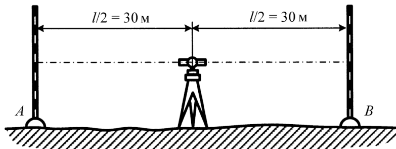
Рисунок Е.1 – Первая конфигурация хода для упрощенной методики испытания
