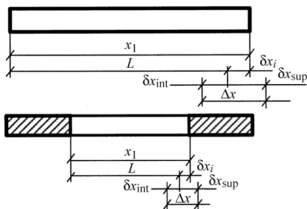
Рисунок 1 – Допуск и отклонение от линейных размеров элементов
