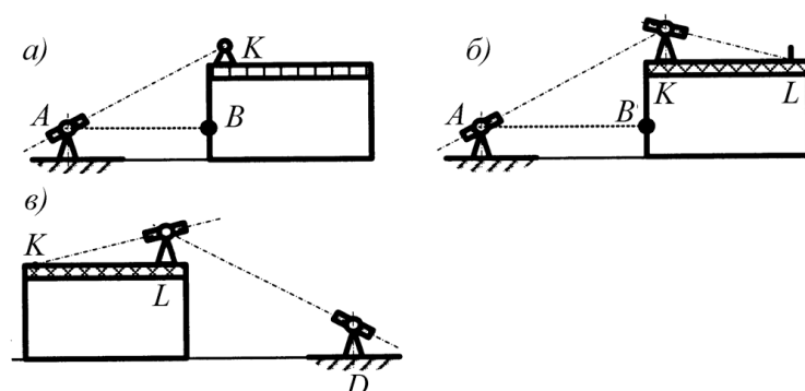
Рисунок Б.7 – Определение положения оси на монтажном горизонте
