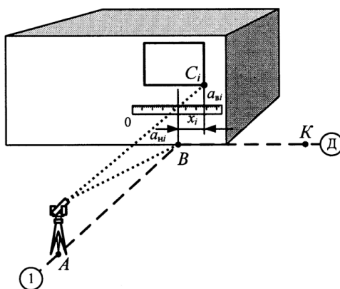
Рисунок В.2 – Метод наклонного проектирования
