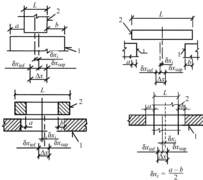
Рисунок 6 – Допуск симметричности и отклонение от симметричности установки элементов
