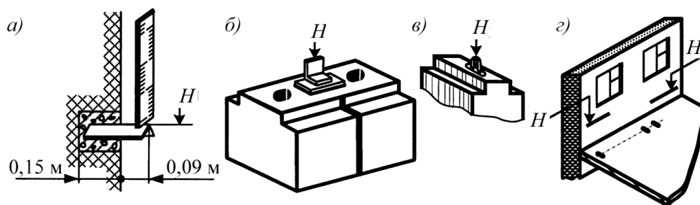
а) – стеной репер в виде угольника; б) – металлическая плашка; в) – монтажная петля; г) – окраска полосы на панели
