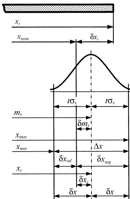
Рисунок Г.2 – Схема взаимосвязи характеристик точности при симметричном распределении геометрического параметра
