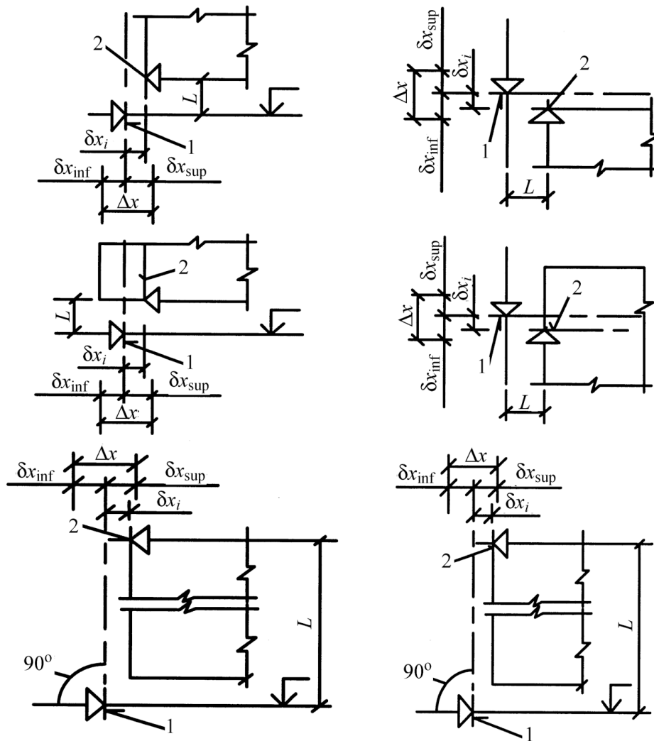
Рисунок 5 – Допуск совмещения и отклонение от совмещения ориентиров
