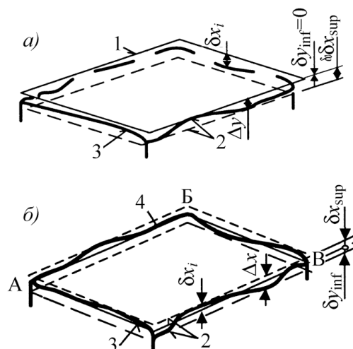
Рисунок 2 – Допуск прямолинейности и отклонение от прямолинейности
