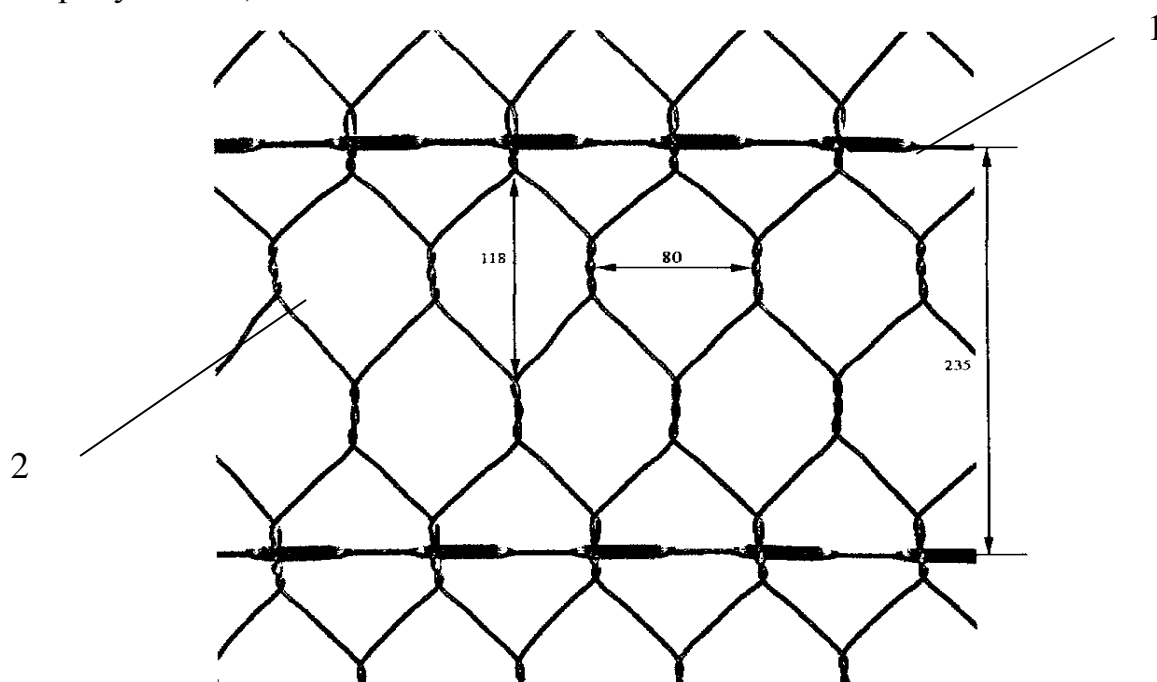
1 - поперечный укрепляющий плоский прут, 2 - ячейка
