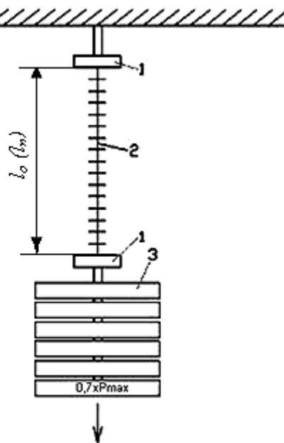
Рисунок Г.5.1. Схема испытания ГМ на длительную прочность
