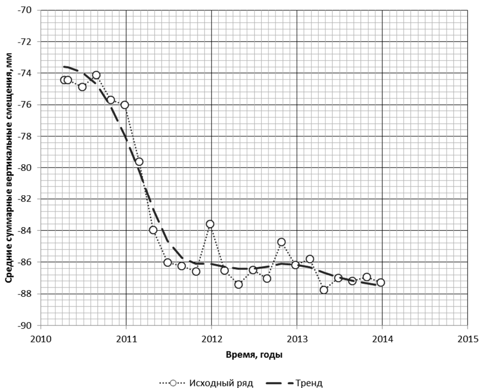
Рисунок Р.2 – График средних суммарных смещений фундаментов
