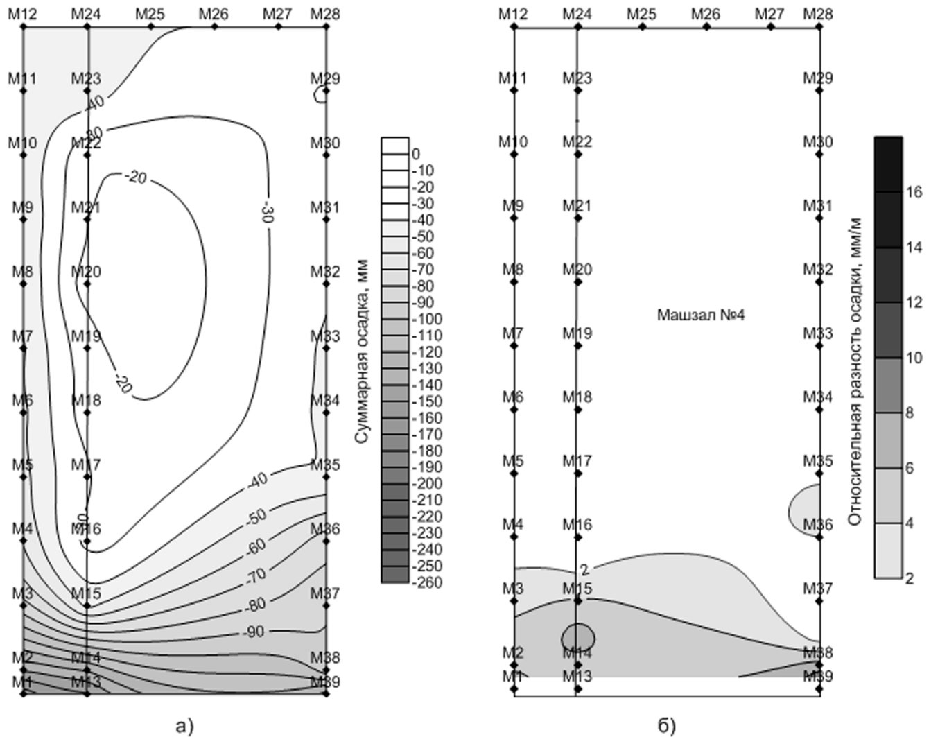
Рисунок Р.7 – Ортогографическая проекция поверхности суммарных вертикальных смещений осадочных марок
