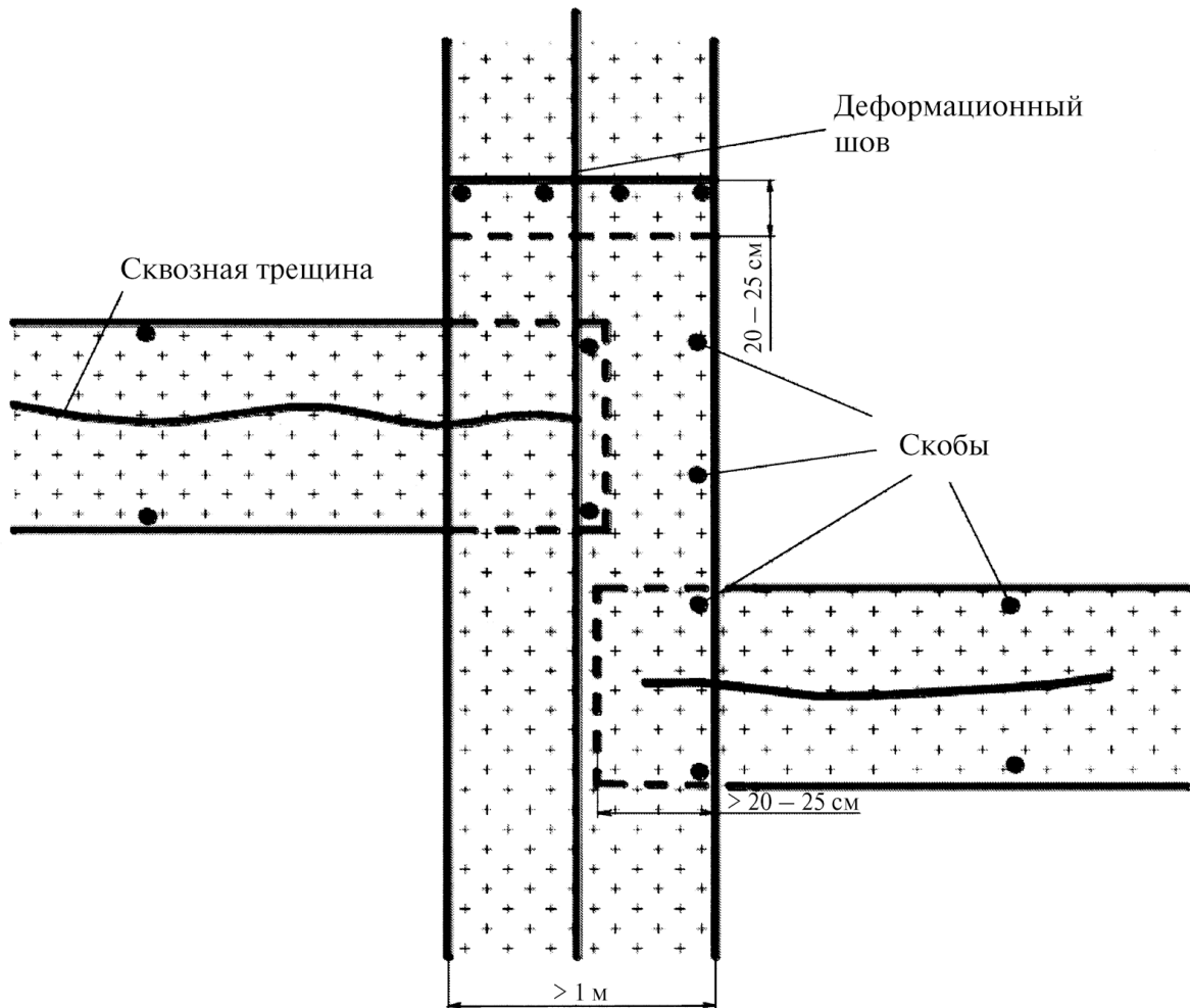
Рисунок 10 – Схема локального армирования геосеткой
