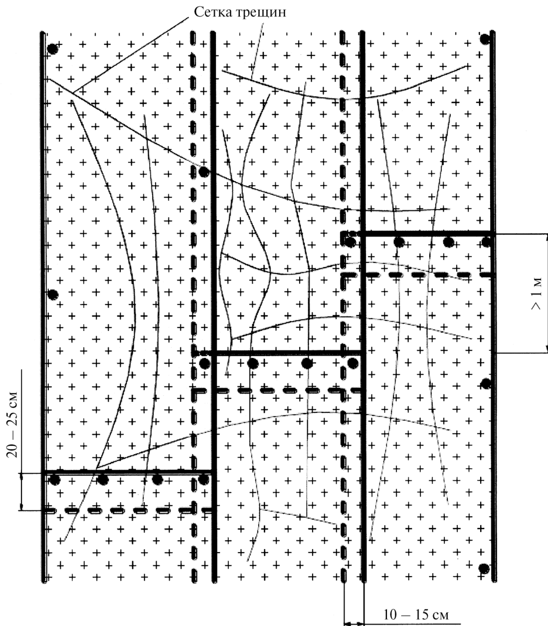
Рисунок 11 – Схема сплошного армирования геосеткой
