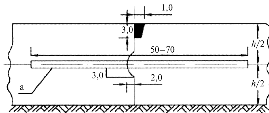
а – штырь-анкер
