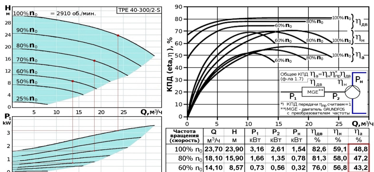
Рисунок В.2 – «Конструктивные» потери КПД насосного агрегата в сборе при ЧРП
