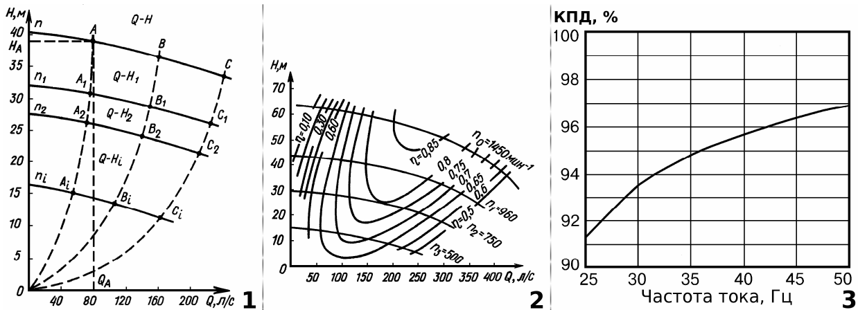
1 – параболы подобных режимов; 2 – универсальная характеристика насоса; 3 – КПД ПЧТ при функциональном изменении частоты выходного тока
