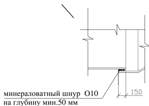
Рисунок 5.1 – Телескопическое соединение газоотводящего патрубка оборудования с газоходом
