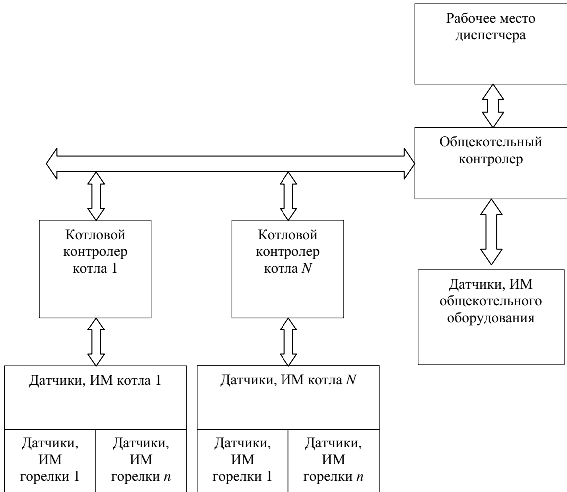
Рисунок Б.2 – Децентрализованная распределенная структура АСУ ОК
