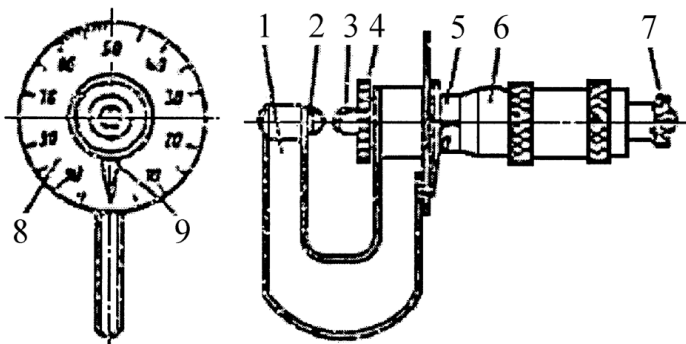
Рисунок Г.7 – Микрометр типа МЛ
