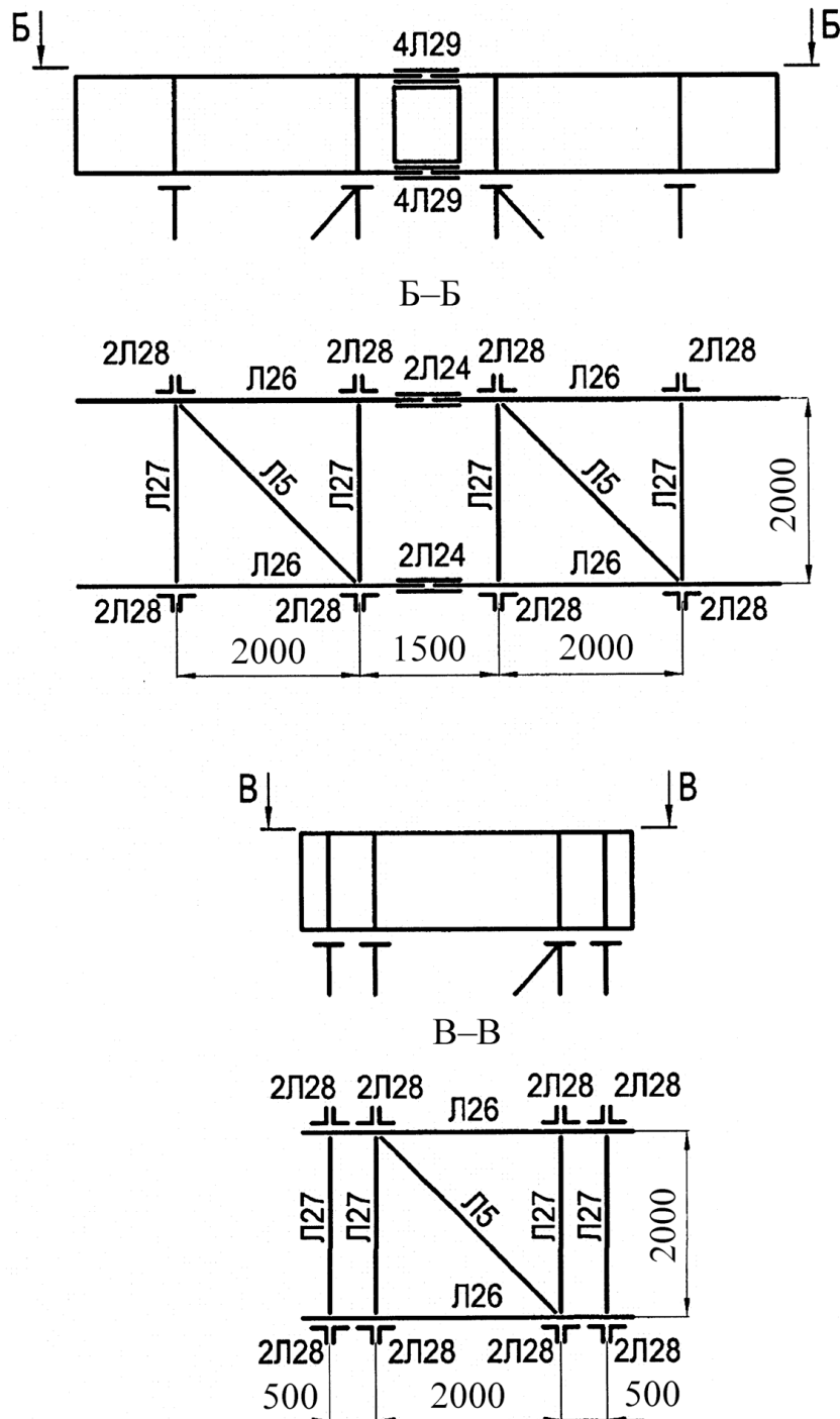
Рисунок А.3 – Примеры компоновки сборных ростверков из инвентарных конструкций МИК-С2
