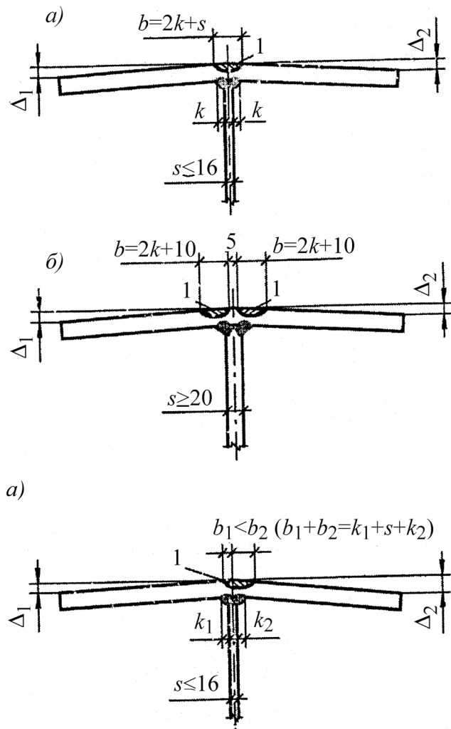
Рисунок И.8, лист 1 – Правка несимметричной грибовидности поясов балок
