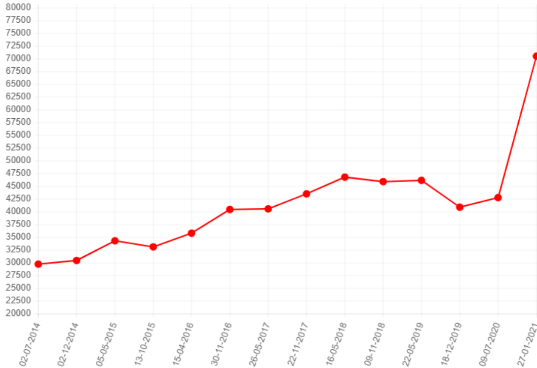
Средний рост цен на металлопрокат
