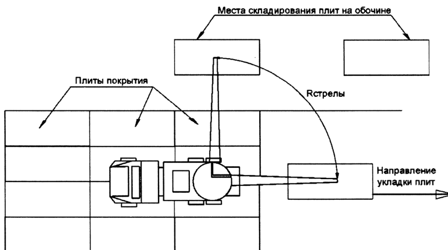
Рисунок 4 – Схема складирования плит на обочине
