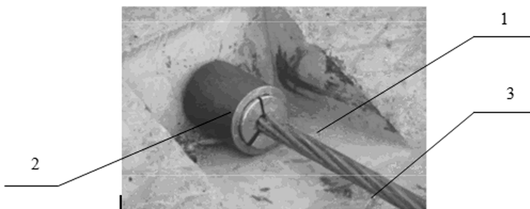
1 – крепежный карман, 2 – анкер, 3 – стальной канат
