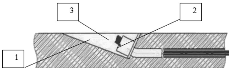
1 – крепежный карман, 2 – анкер, 3 – обрезанный стальной канат
