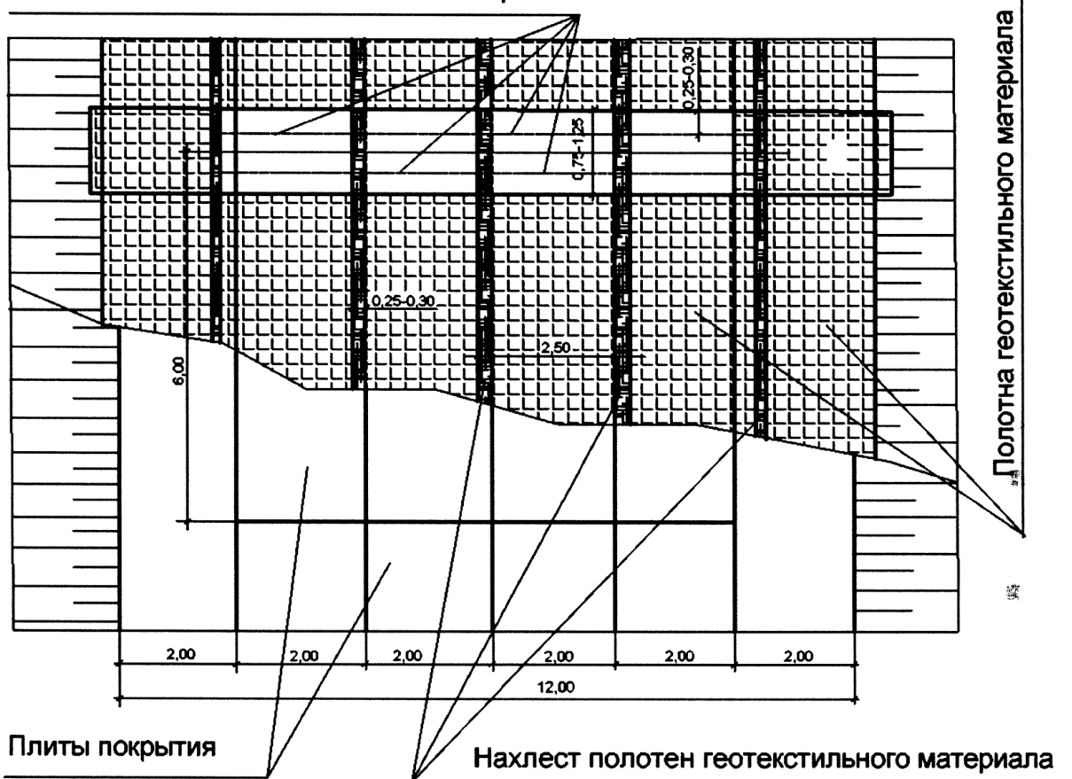
Рисунок 10, лист 1– Вариант раскладки геотекстильного материала
