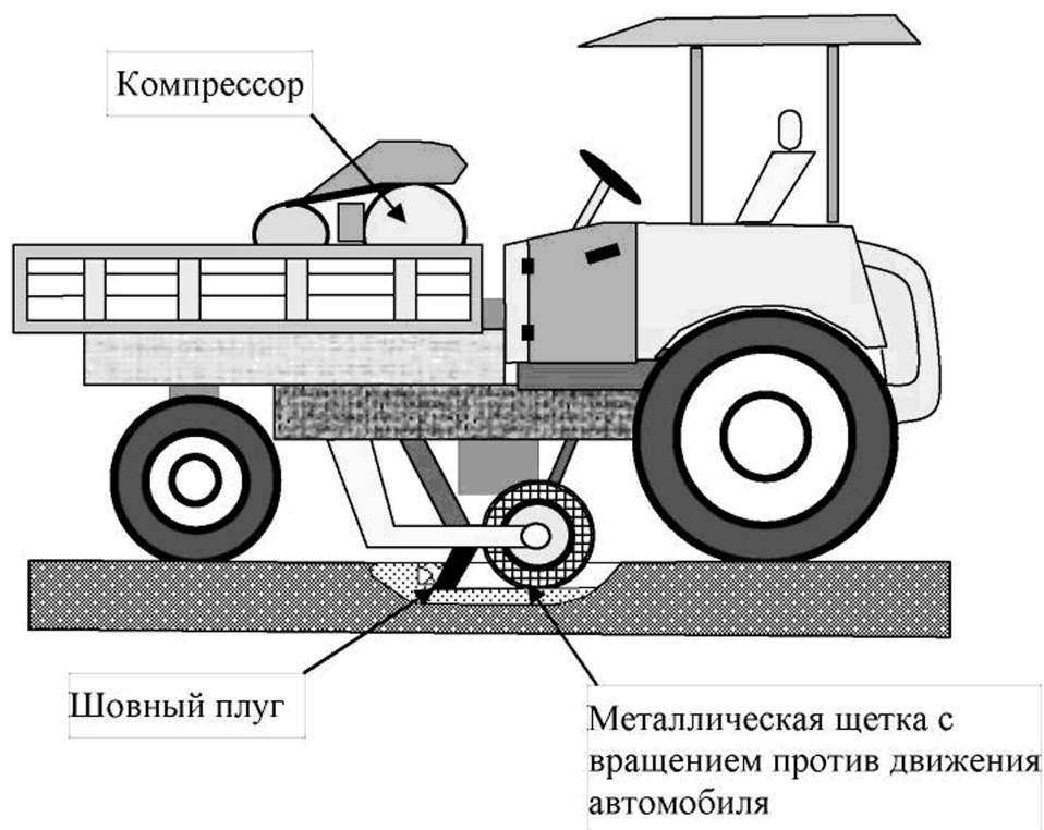
Рисунок 14 – Вариант щеточной машины оборудованной шовным плугом
