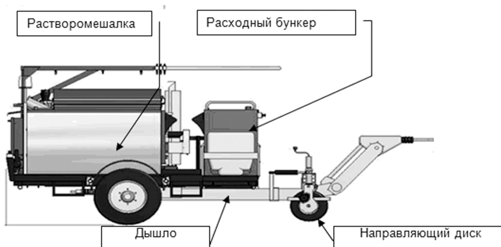
Рисунок 13 – Вариант конструкции заливщика шва
