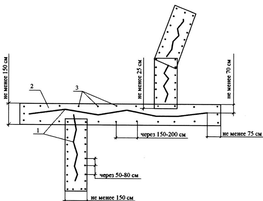
1 – продольные и поперечные трещины; 2 – полосы трещинопрерывающей (армирующей) прослойкой; 3 – дополнительная фиксация полос
