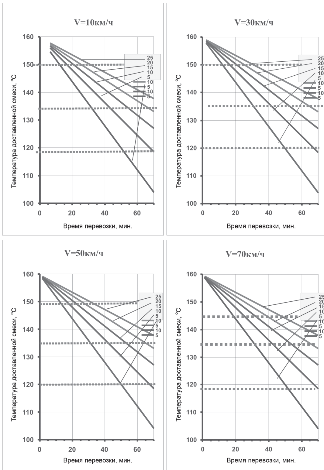
Рисунок В.1 – Время перевозки горячей асфальтобетонной смеси в автомобилях самосвалах (при температуре отгрузки t_{\text{нач}} = 160 \text{ }^\circ\text{C} )
